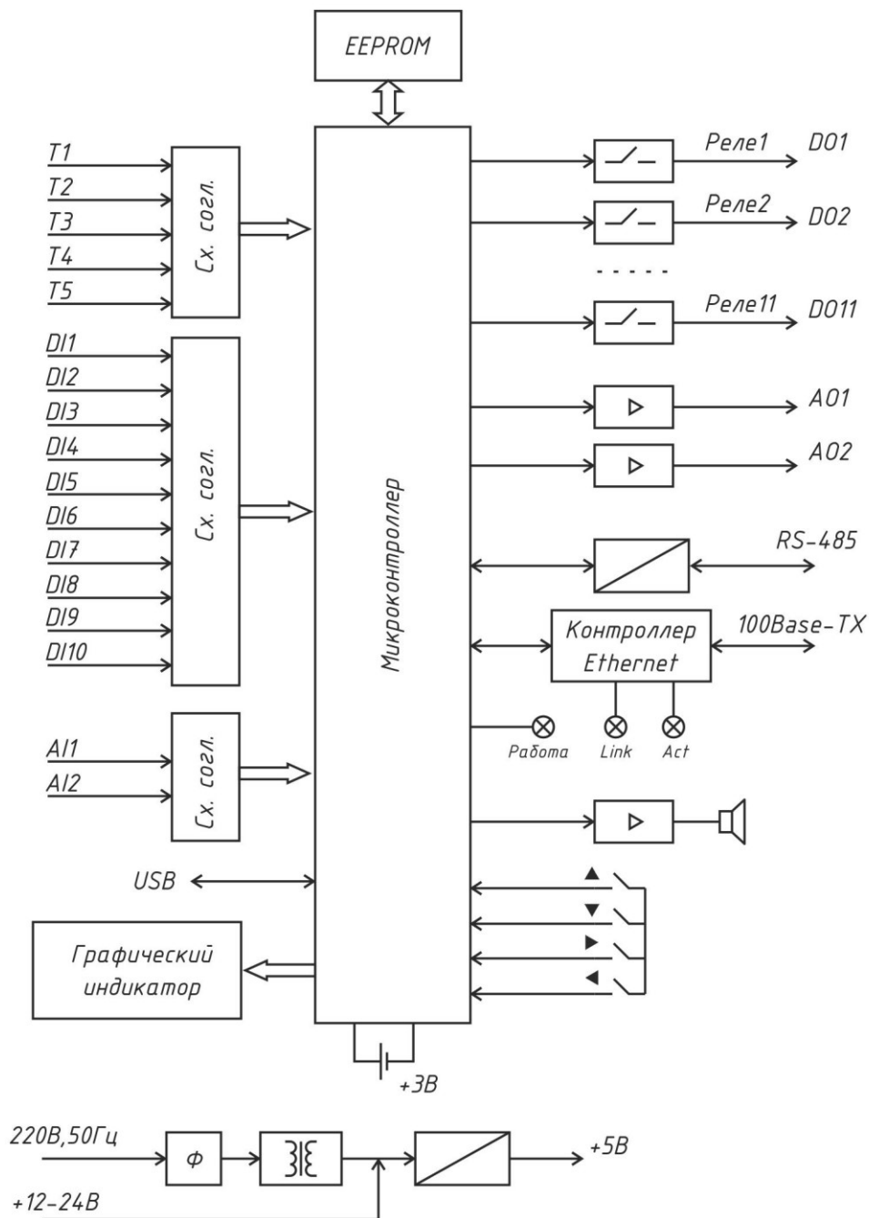
Рисунок 4 – Структурная схема контроллера «Saturn-PLC»
